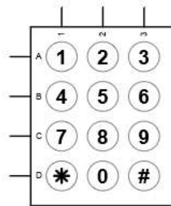
Fig. 7.Matrix Keypad.
